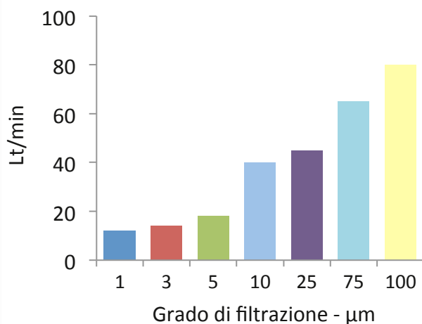
Portata (acqua, 10", \Delta p 0,1 bar)
